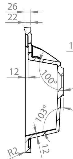
PRZEKRÓJ G-G SKALA 1 : 9
