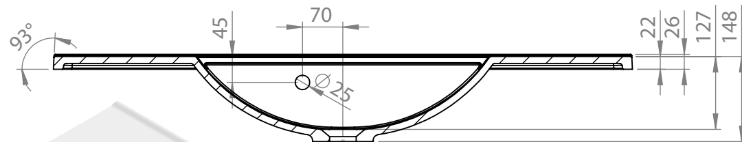
PRZEKRÓJ H-H SKALA 1 : 9
